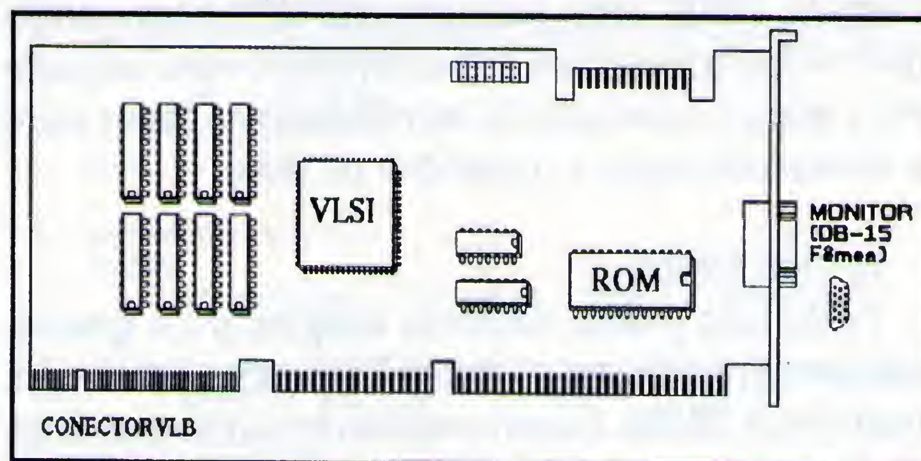
Figura 12 - placa SVGA de 32 bits (VLB)
